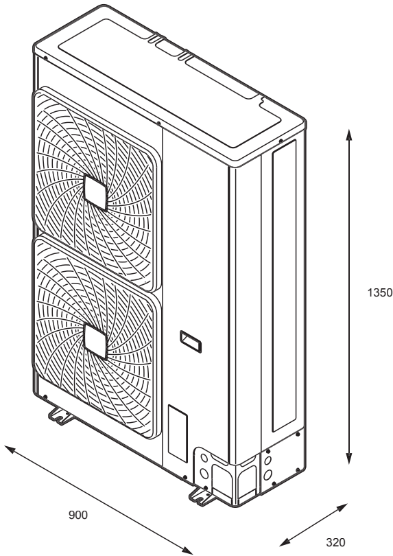
Dimensiones MiniZeas
